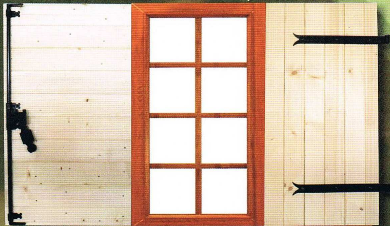
N° 4 Volet 2 plis croisés Lames extérieures verticales épaisseur 27mm Lames intérieures horizontales épaisseur 16 mm
