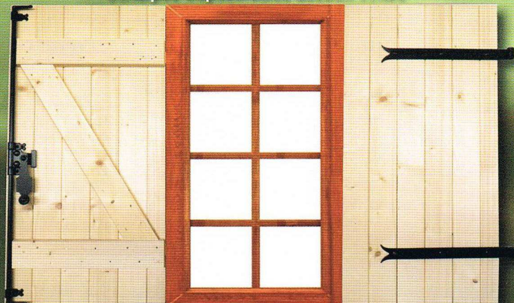
N° 1 Volet barres et écharpes Barres trapézoïdales section 20x95 écharpes trapézoïdales section 17x95
