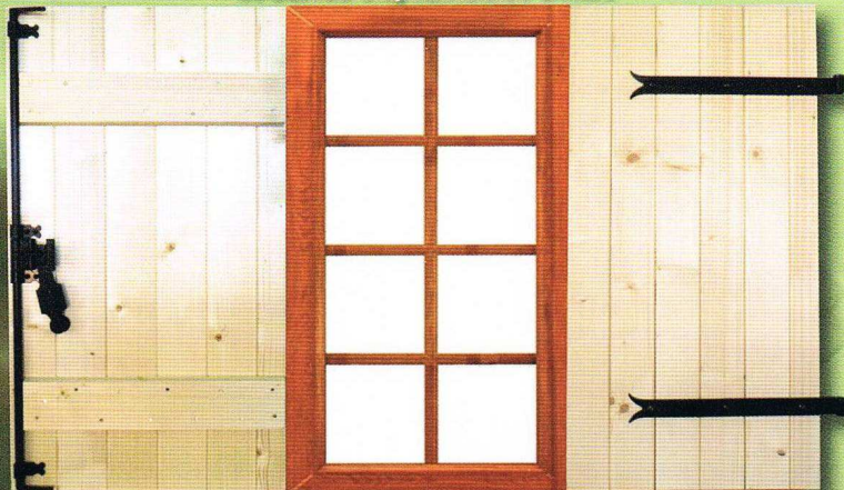
N° 2 Volet clés barres Clés métalliques bichromatées Ø 8 et barres trapézoïdales 20x95
